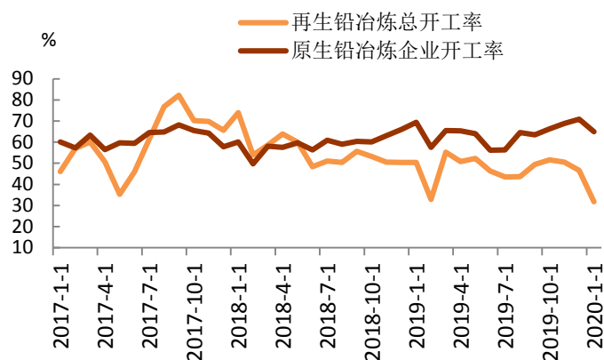
图表 10 冶炼厂开工情况
